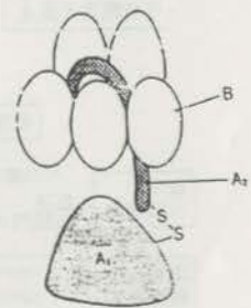
ベロ毒素の構造
